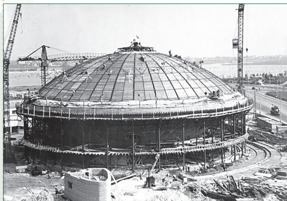
Строительство Казанского цирка. 1960-е годы
